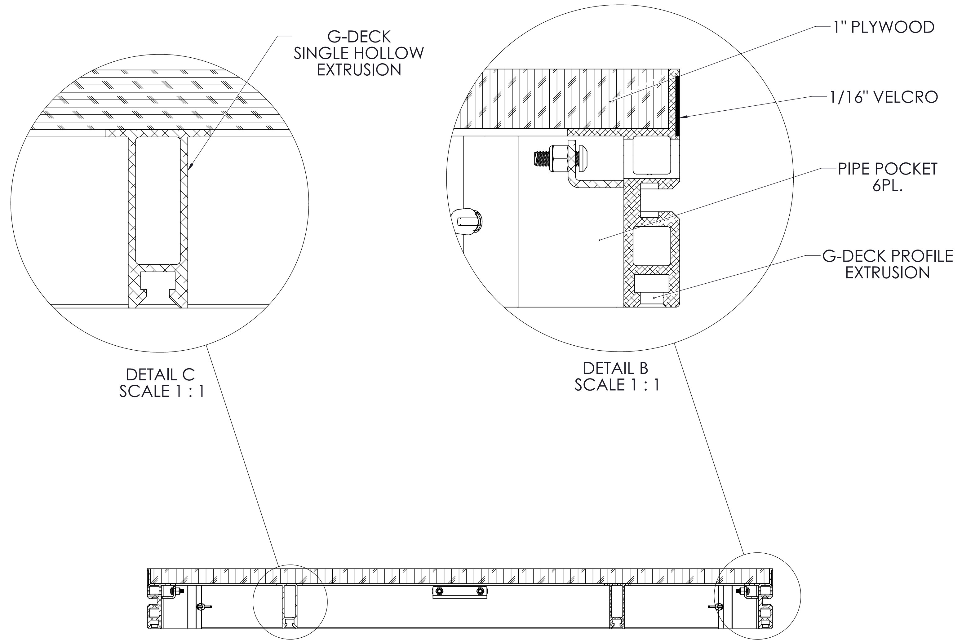
SECTION A-A SCALE 1 : 4
