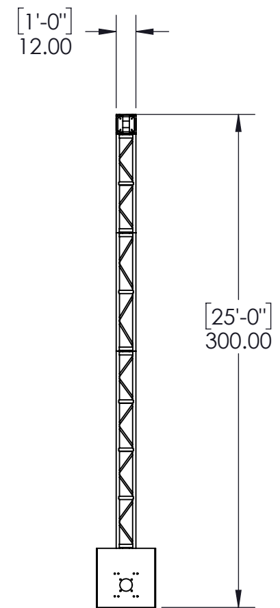
END ELEVATION
